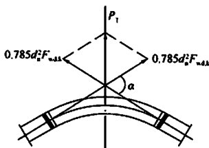
图 4.5.2-1 管道水平方向 弯头推力图
